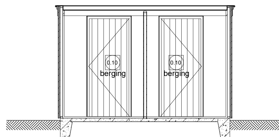
Doorsnede K
