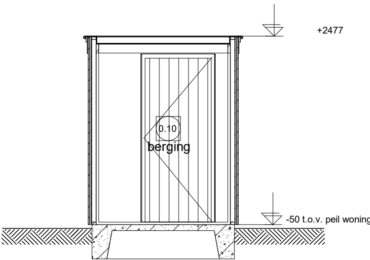
Doorsnede H
