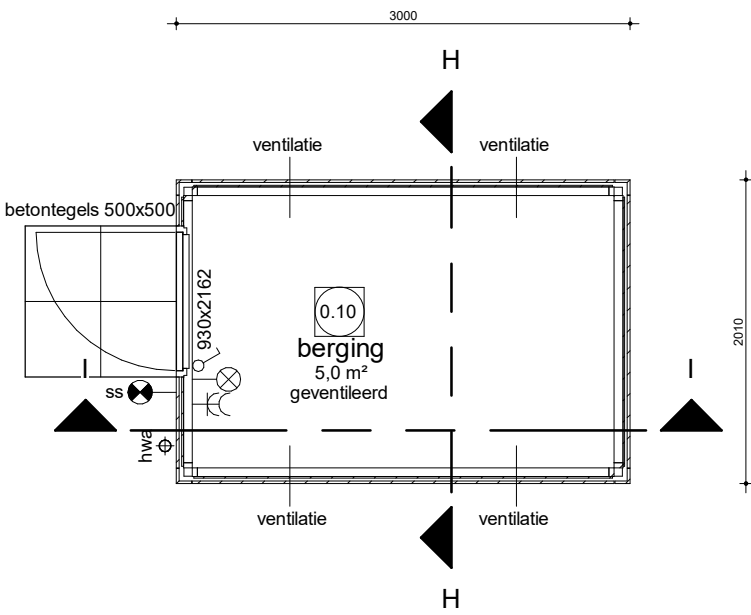
Begane grond
