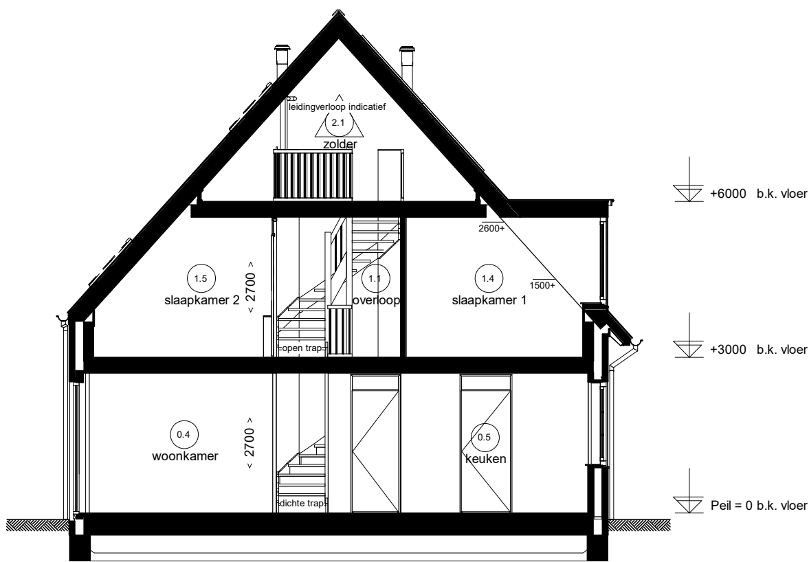
Doorsnede 19.1
