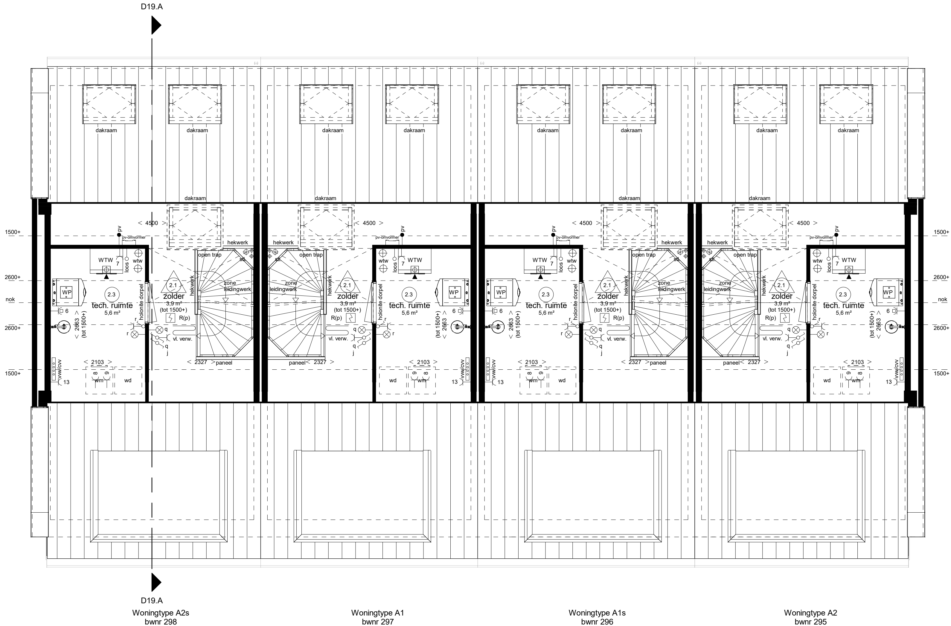
Tweede verdieping
