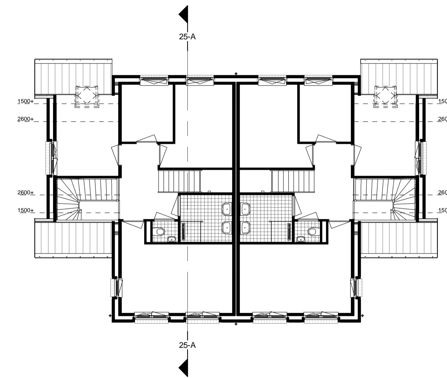
Eerste verdieping Type H3 bwnr. 169 Type H3s bwnr. 170
