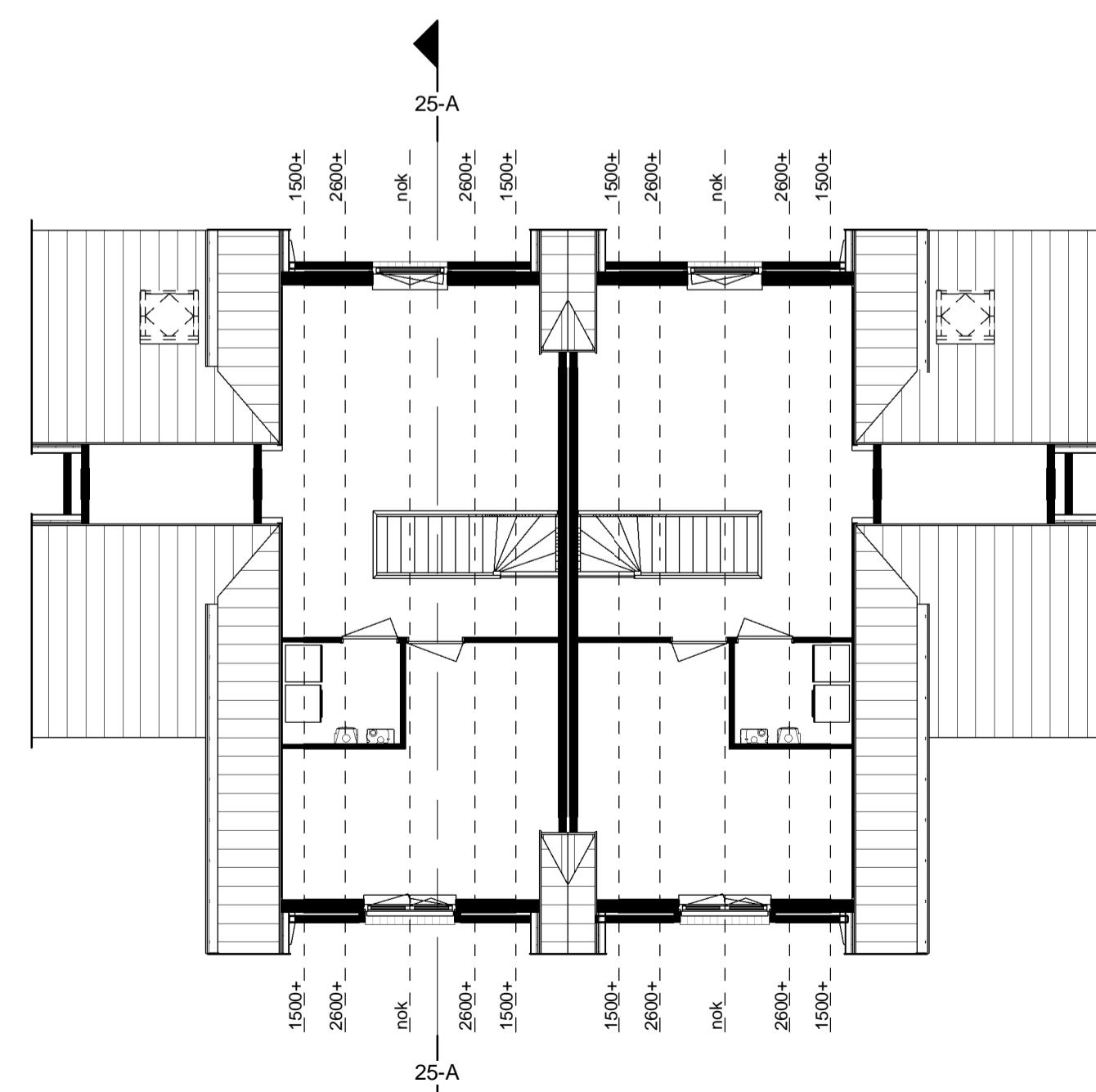
Tweede verdieping Type H3 bwnr. 169 Type H3s bwnr. 170
