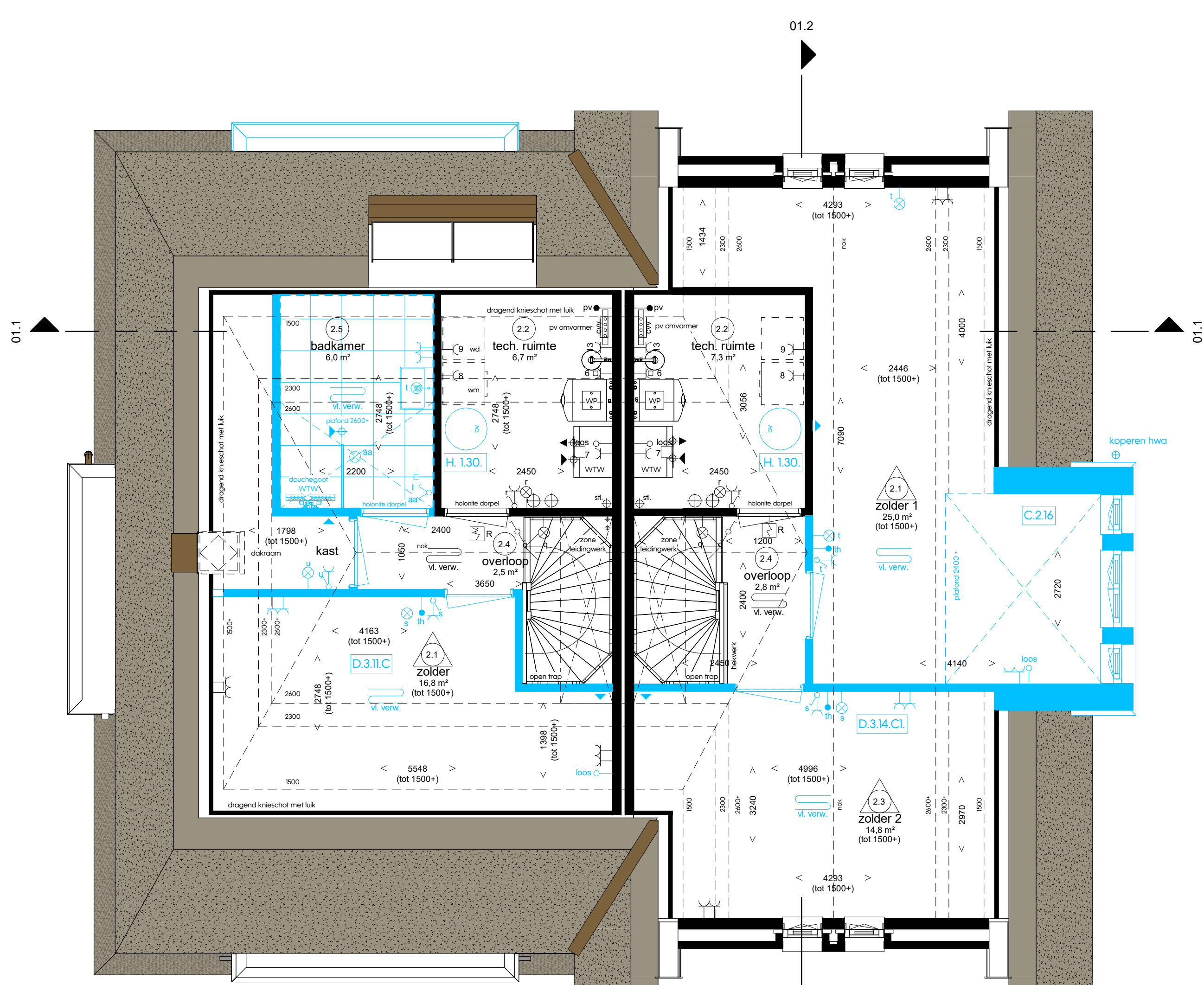
Tweede verdieping
