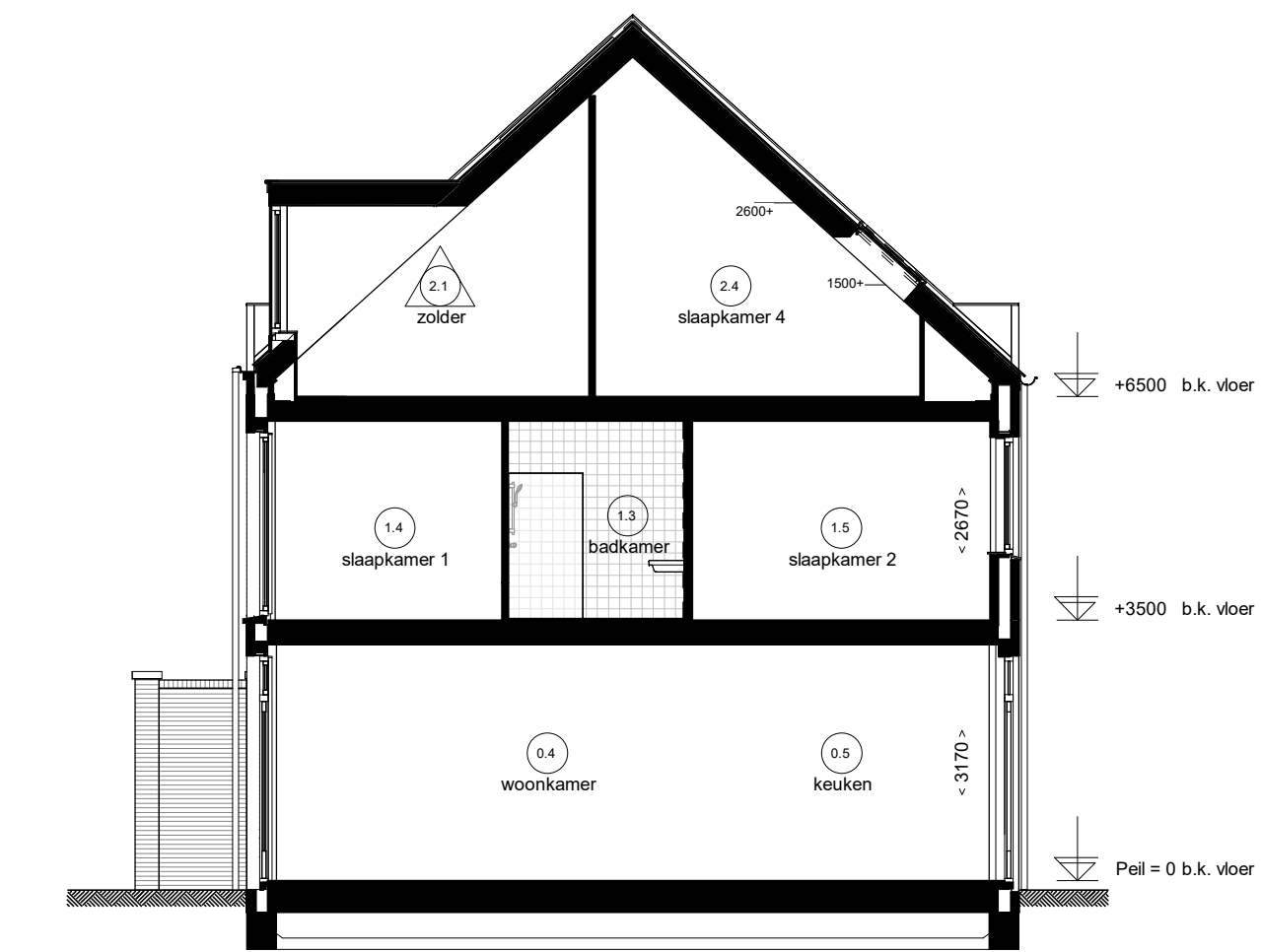
Doorsnede D14.A
