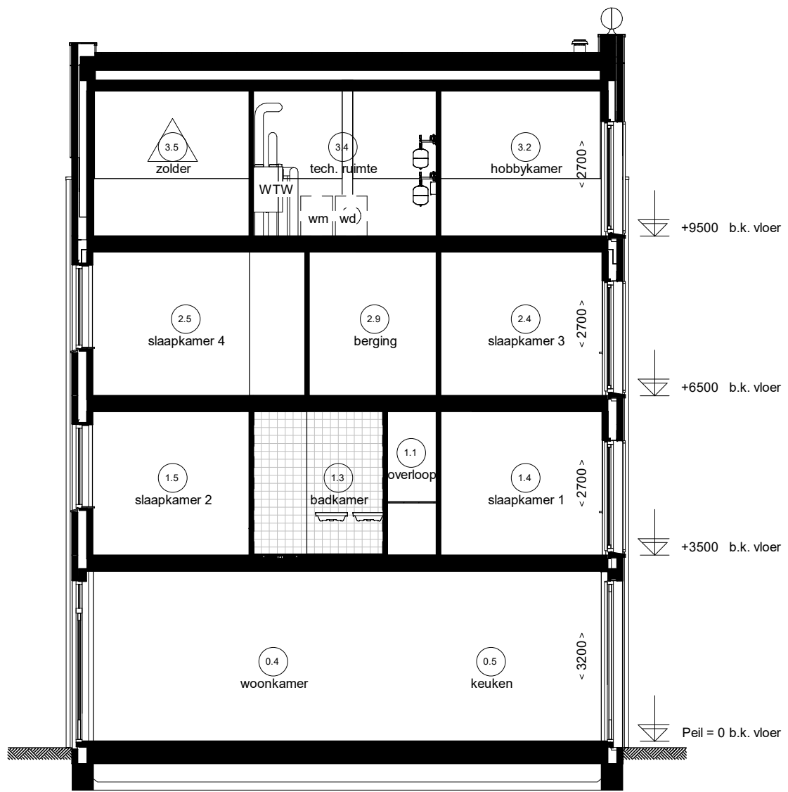
Doorsnede D14.C
