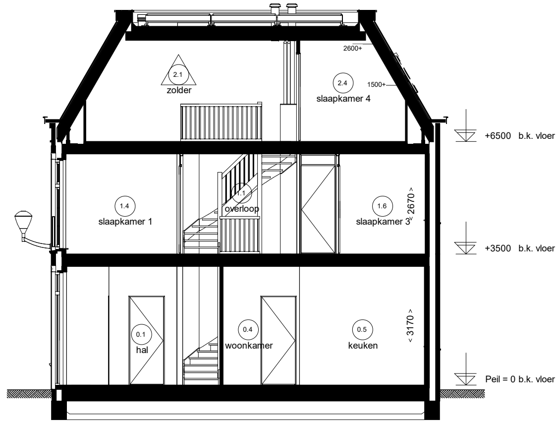
Doorsnede D14.B
