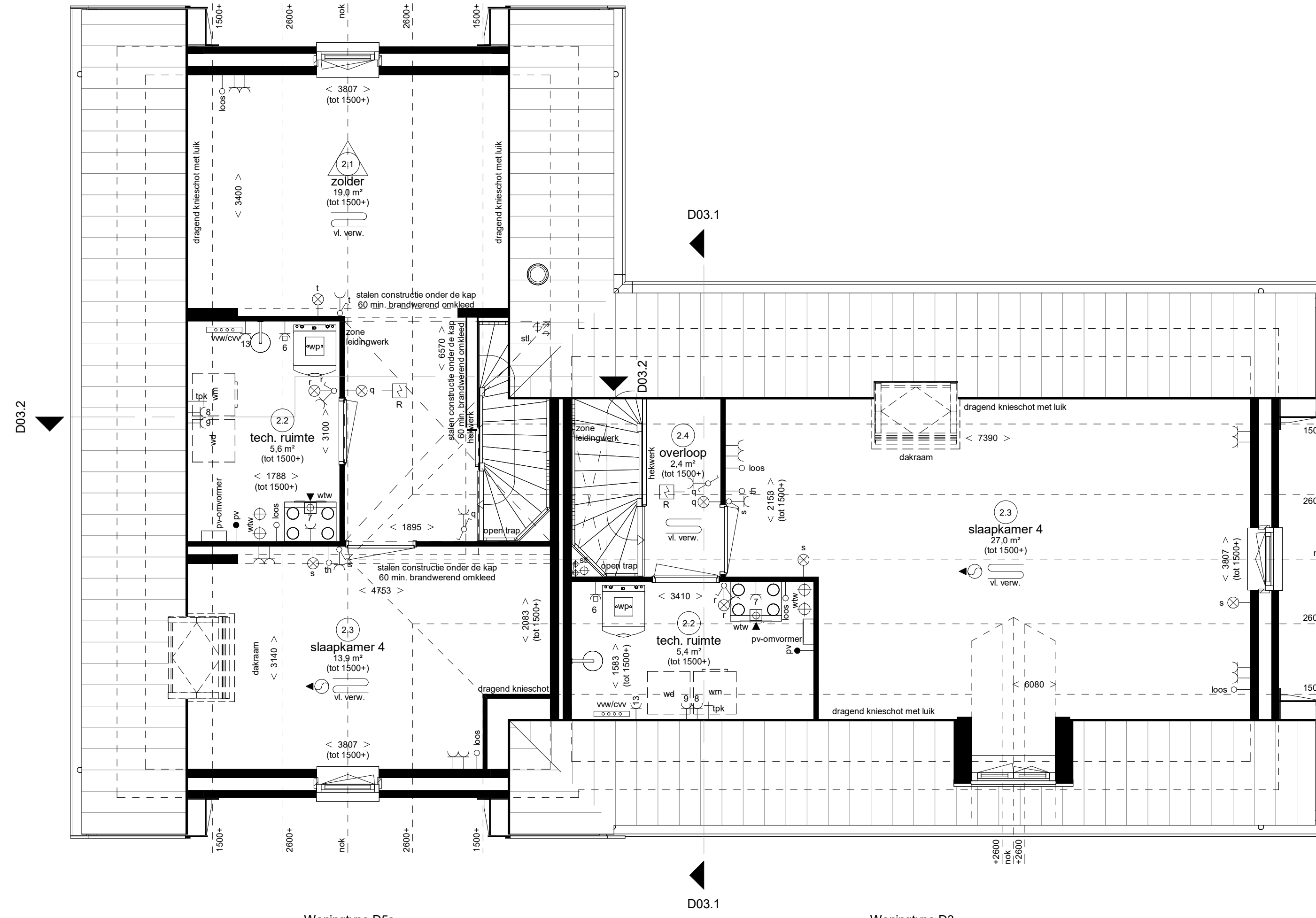
Woningtype D5s bwnr 320 Woningtype D3 bwnr 319 Tweede verdieping
