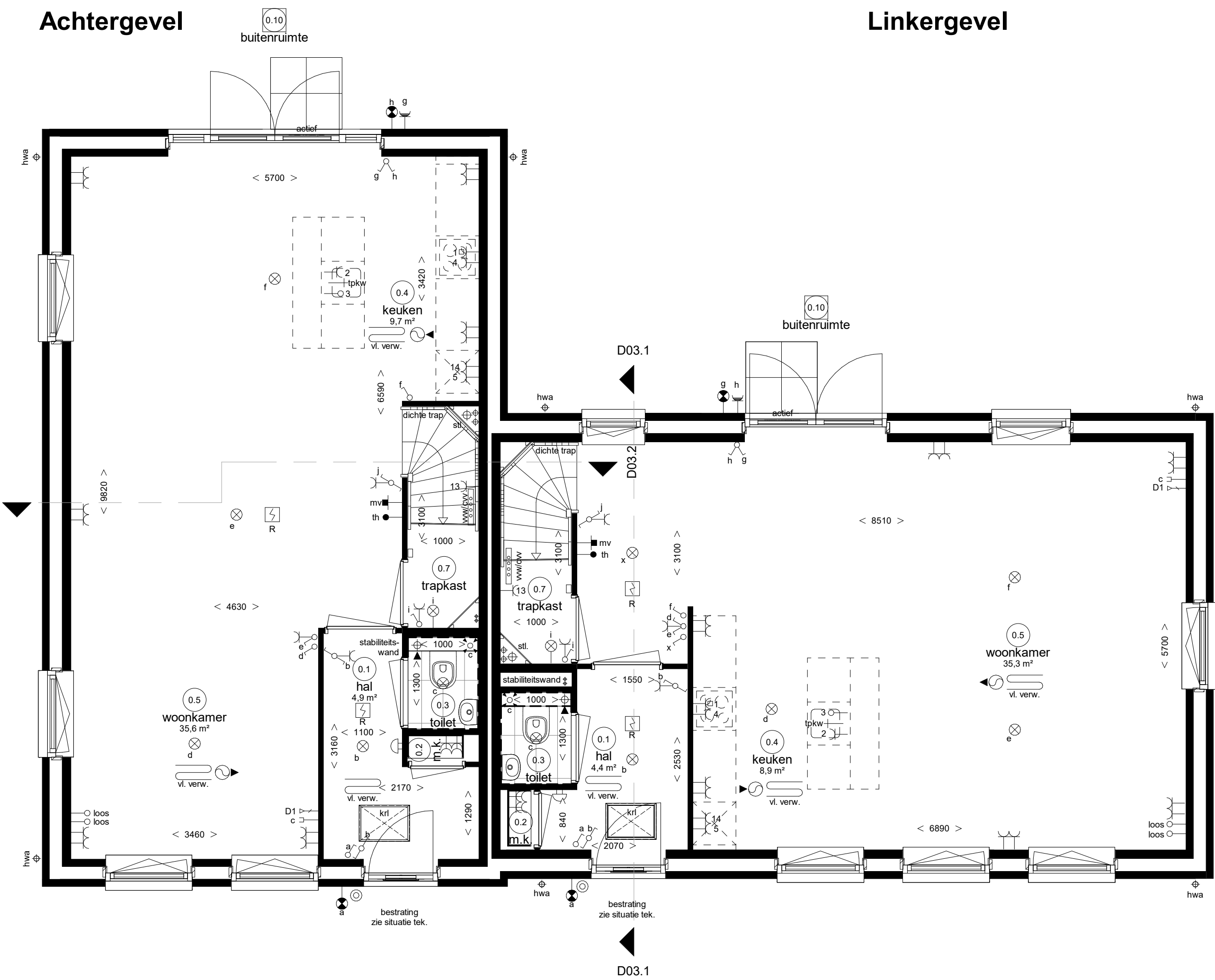
Woningtype D5s bwnr 320 Woningtype D3 bwnr 319 Begane grond
