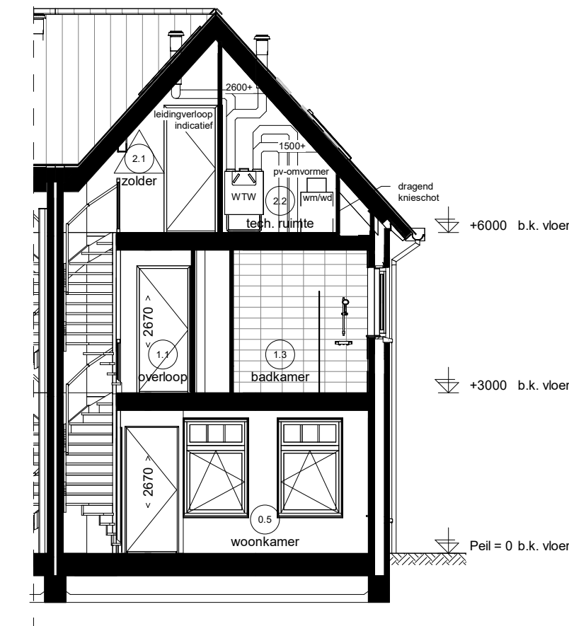
Doorsnede D03.2
