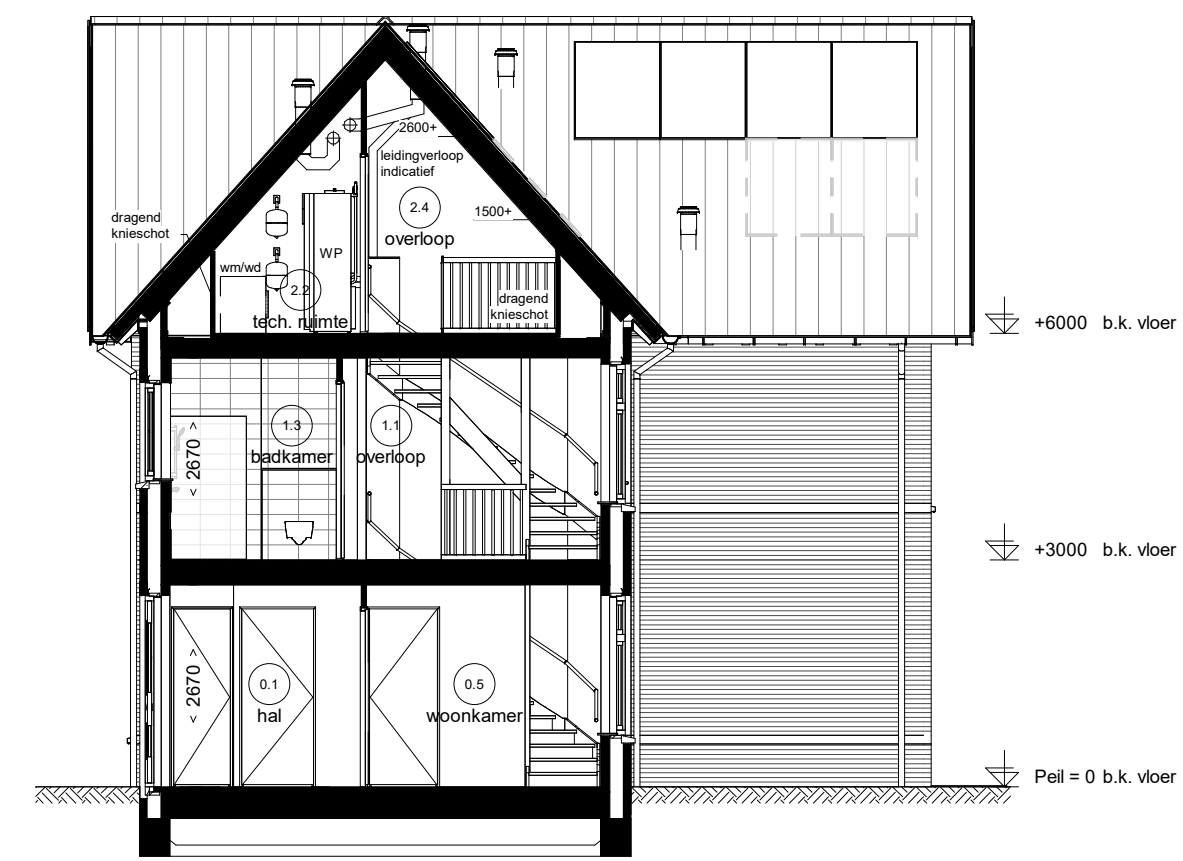
Doorsnede D03.1
