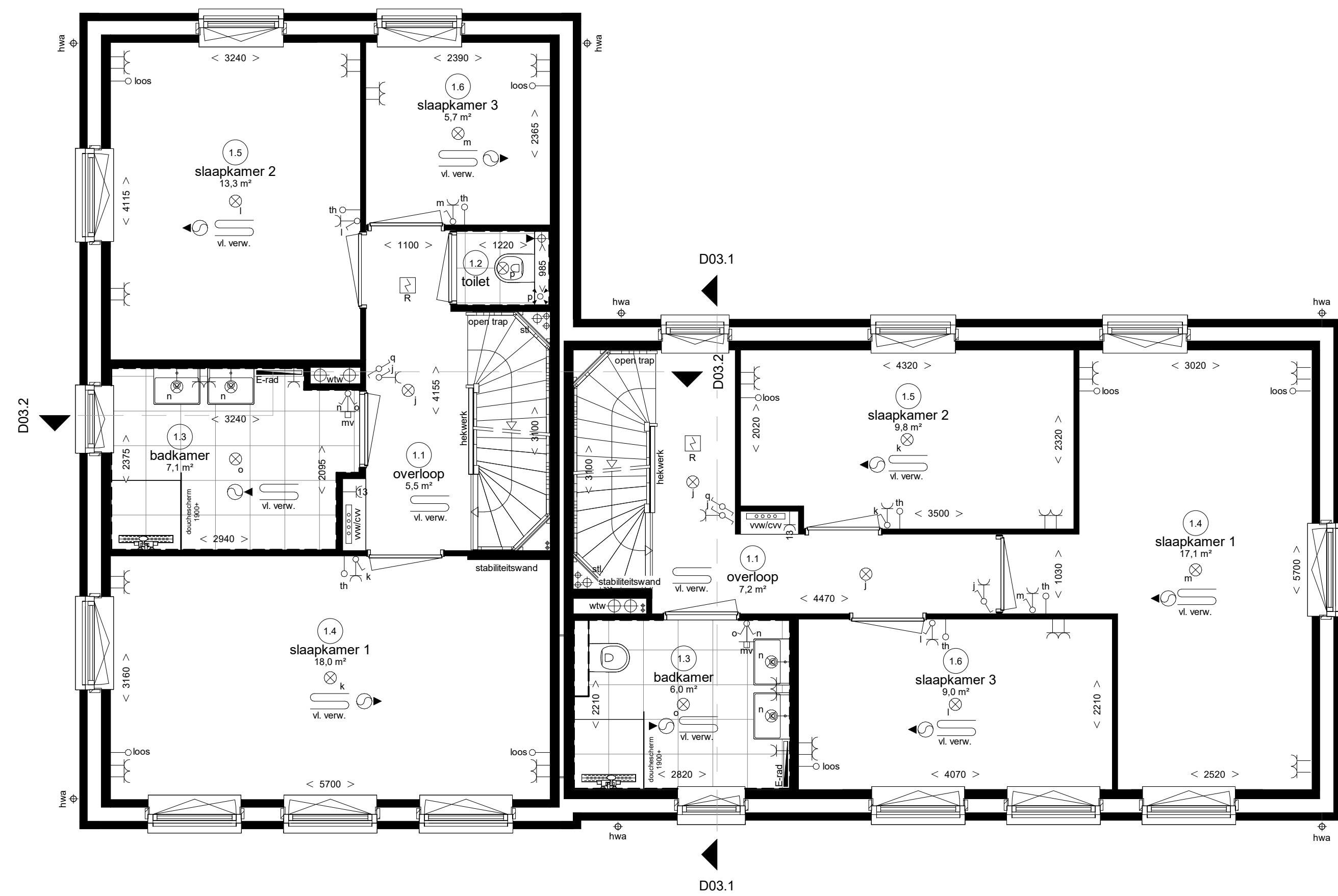
Woningtype D5s bwnr 320 Woningtype D3 bwnr 319 Eerste verdieping
