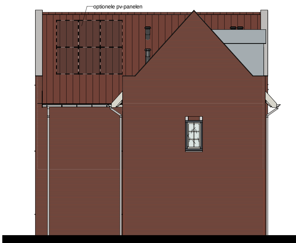
Linkergevel
