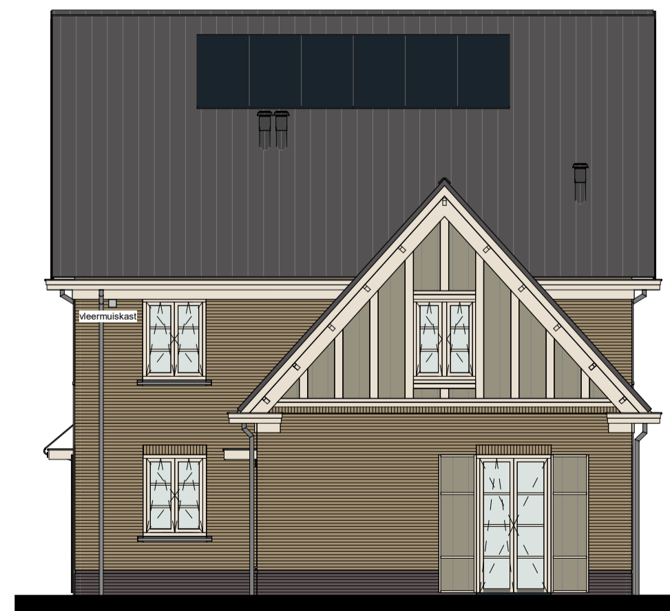
Woningtype HWs (Hoogerwerf S) bwnr 150
