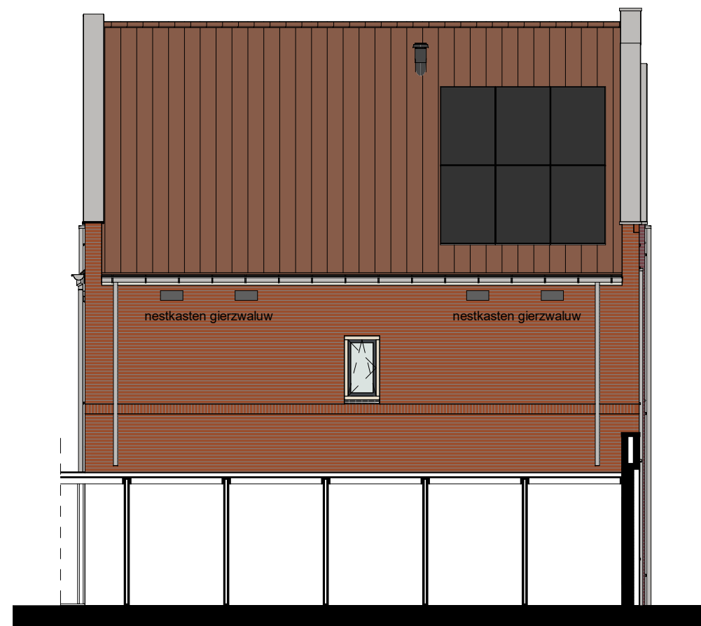
Linkergevel
