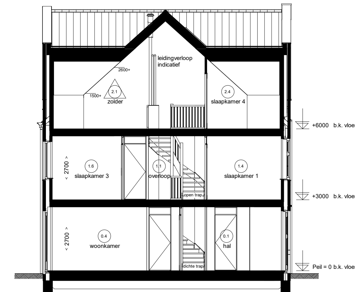
Doorsnede D7.D
