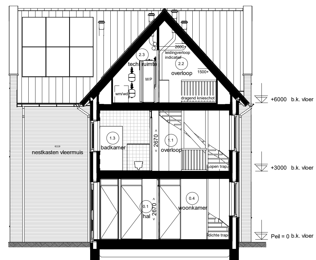
Doorsnede D7.B
