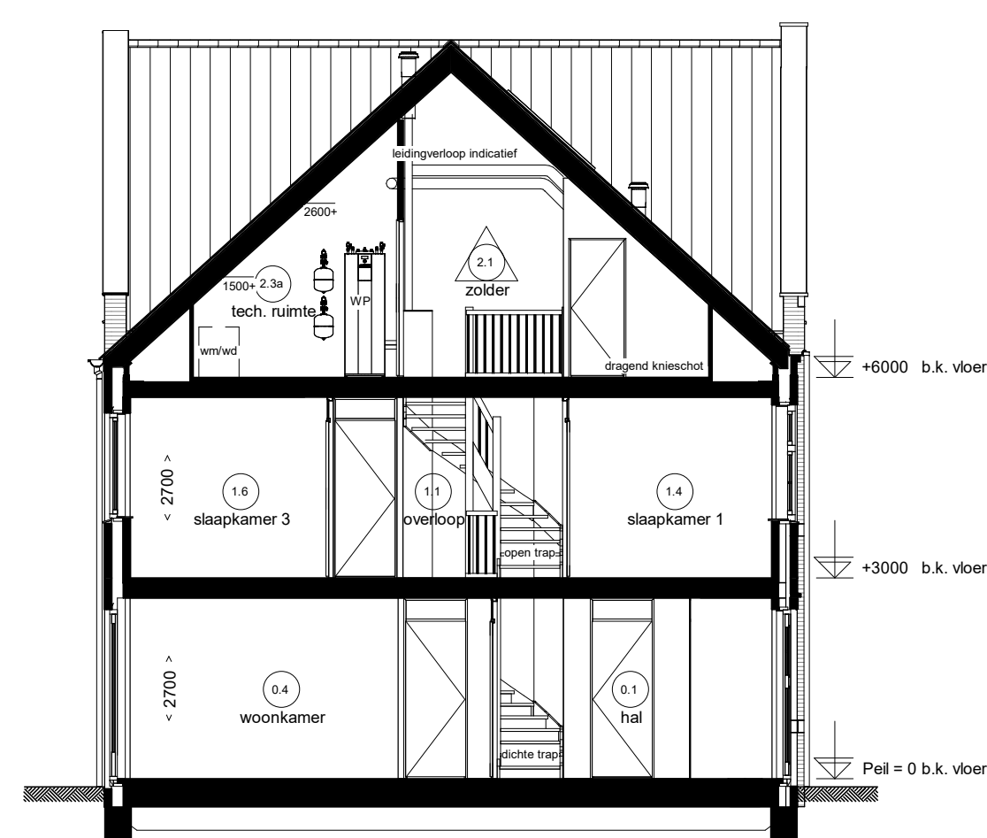
Doorsnede D7.A
